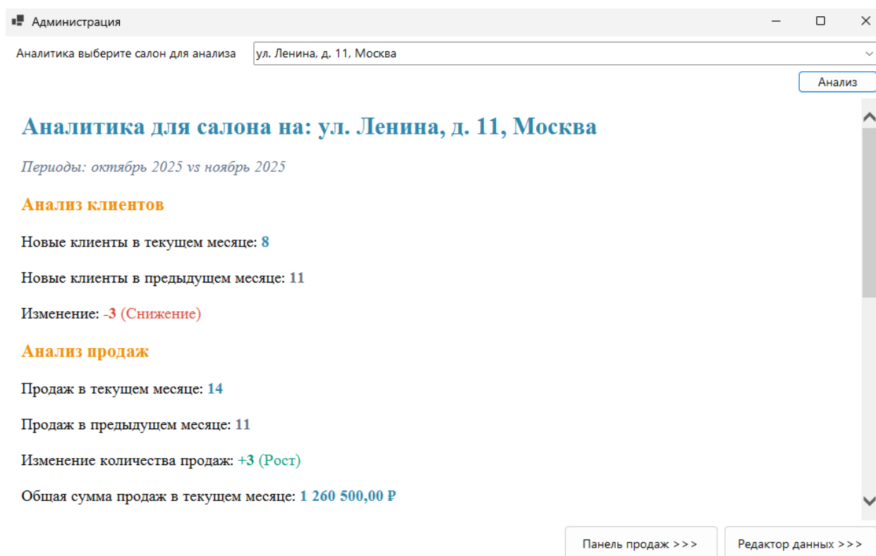
Рисунок 3.2 Окно администратора
