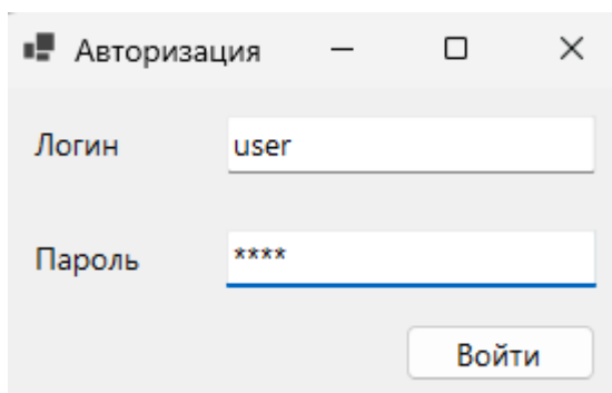
Рисунок 3.1 Окно авторизации
